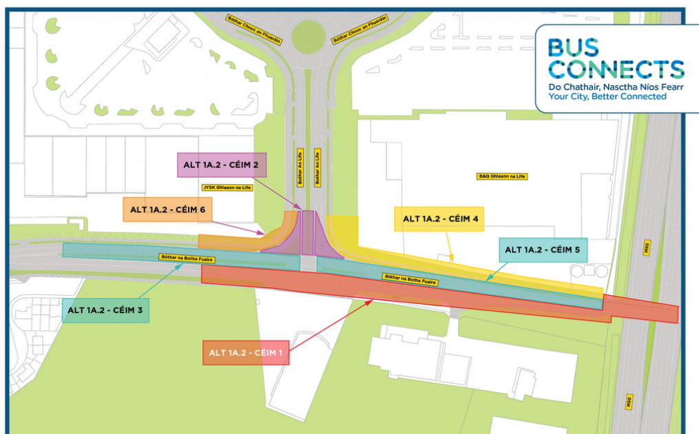
Fig1: Limistéar oibre agus céimeanna tógála (Céimeanna 1-6)
